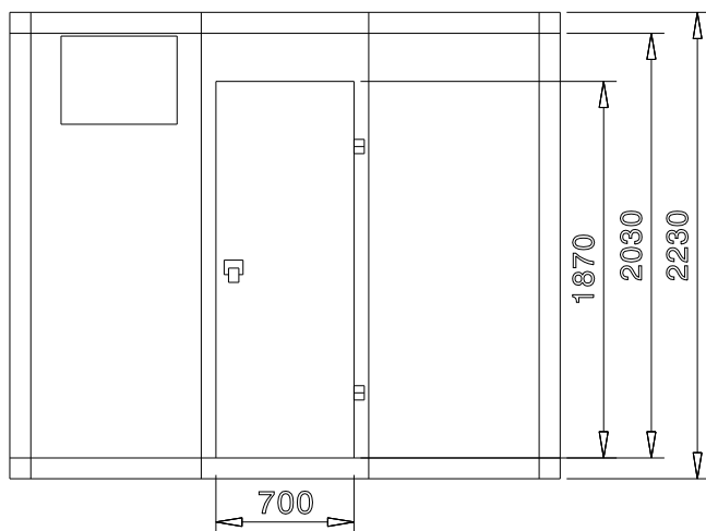
Zij aanzicht
